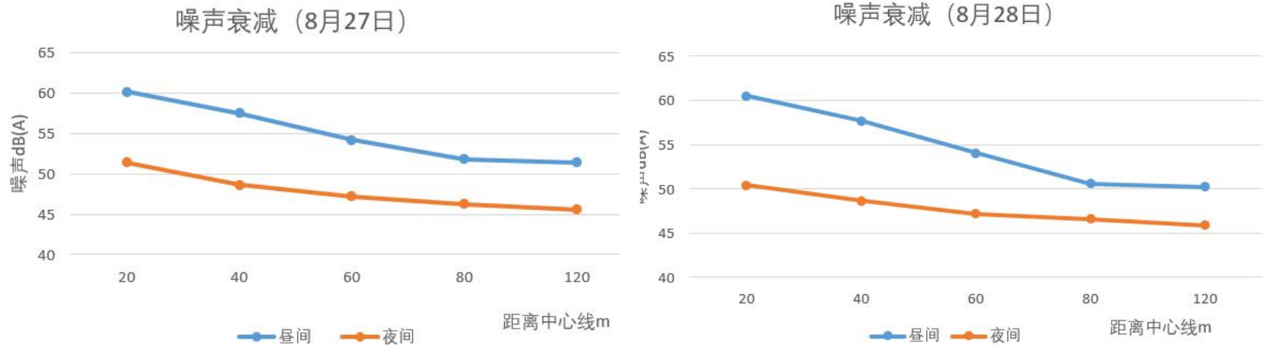
图 7.3-2 噪声衰减断面昼间和夜间噪声衰减曲线
